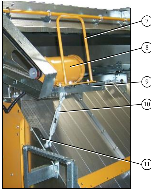
Top Auger motor and motor mount.
